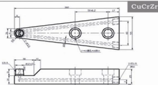
三角握杆 HD-54
